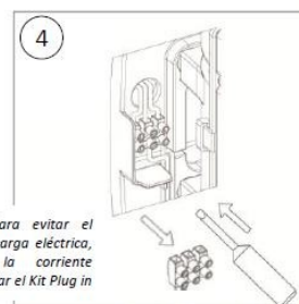
Desconectar los cables y quitar la regleta
